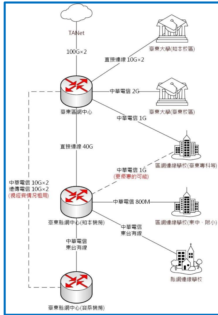
網路架構圖(規劃)
