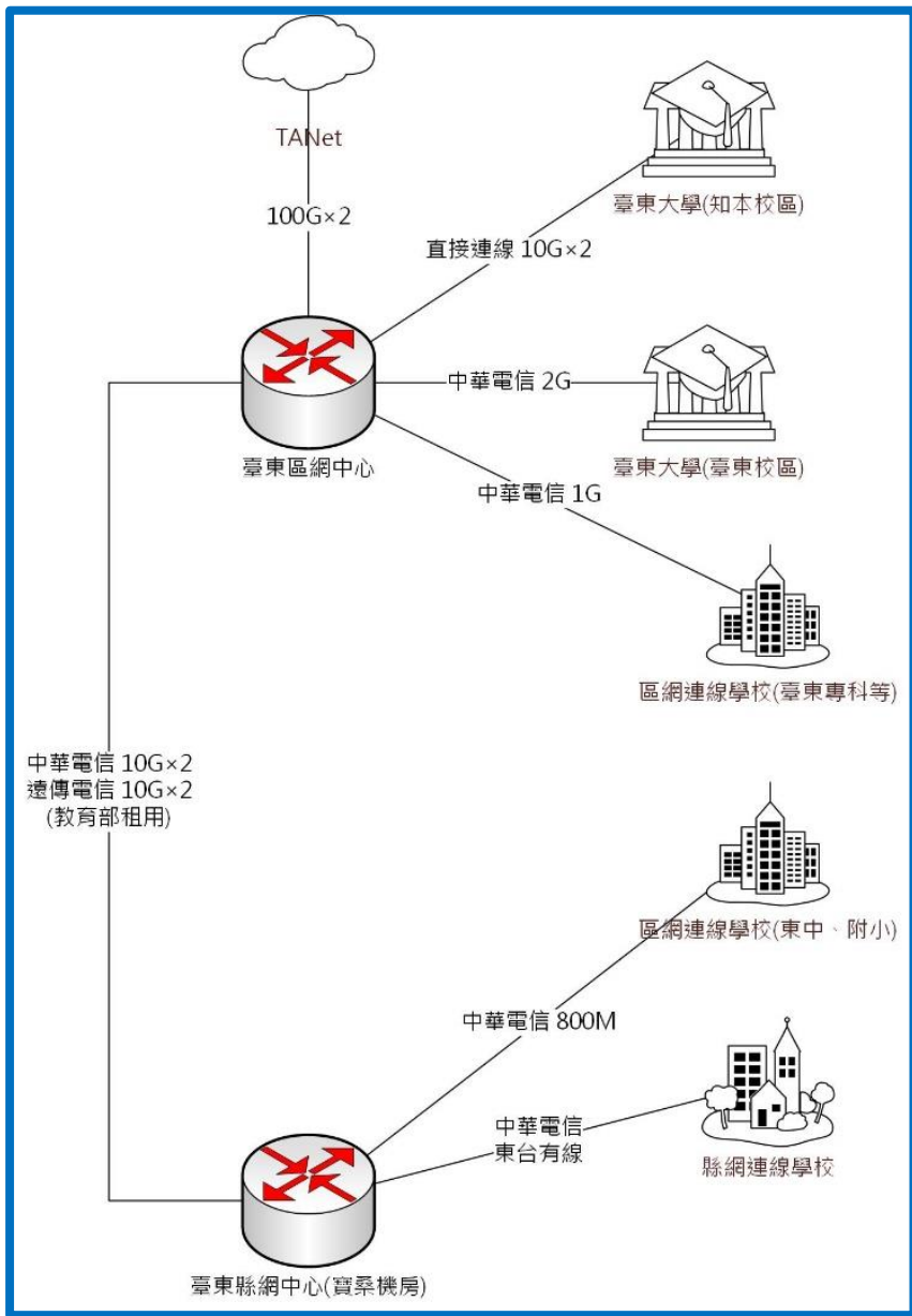
網路架構圖(現況)
