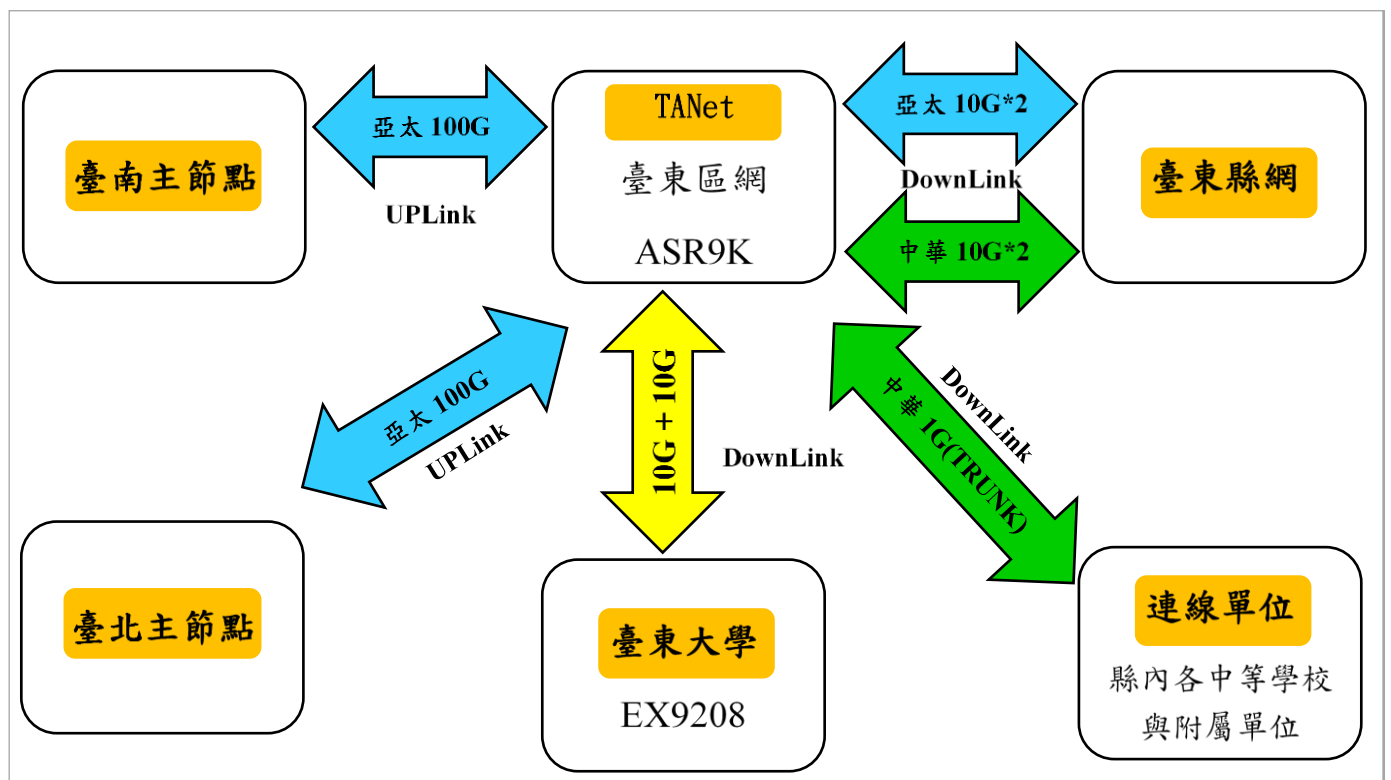
圖 2 臺東區網中心與連線單位網路示意圖
