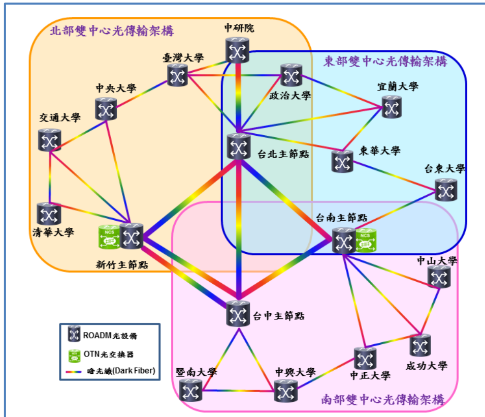
圖 1 臺東區網中心（臺東大學）與 TANet 光纖網路架構圖
